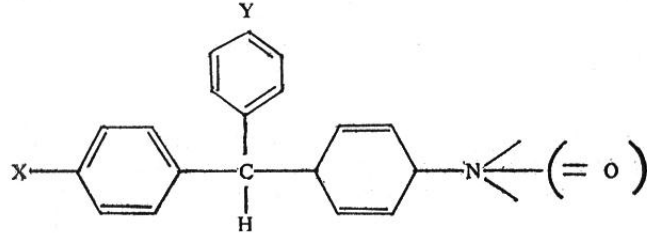
ट्राय फेनिल मिथेन रंग गटाचा एक सर्वसाधारण सांगाडा
