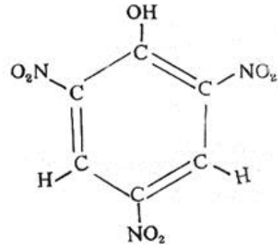
ट्राय नायट्रो फेनॉल (टी.एन.पी. किंवा पीक्रिक ॲसिड) स्फोटक
