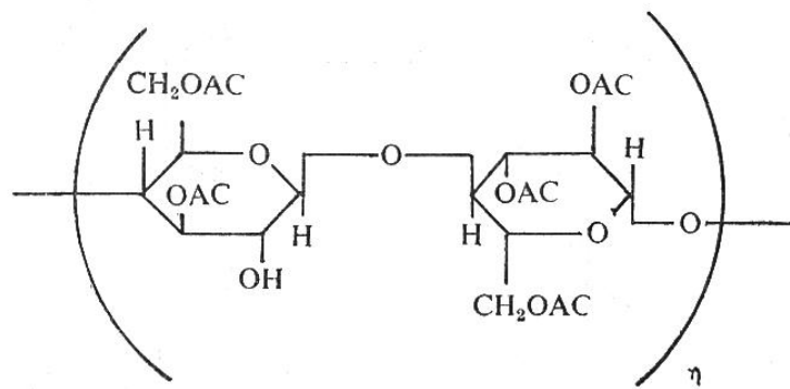
सेल्युलोज अॅसिटेट प्लॅस्टिकची रेणुरचना
