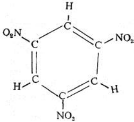
ट्राय नायट्रो बेन्झीन (टी.एन.बी.) स्फोटक
