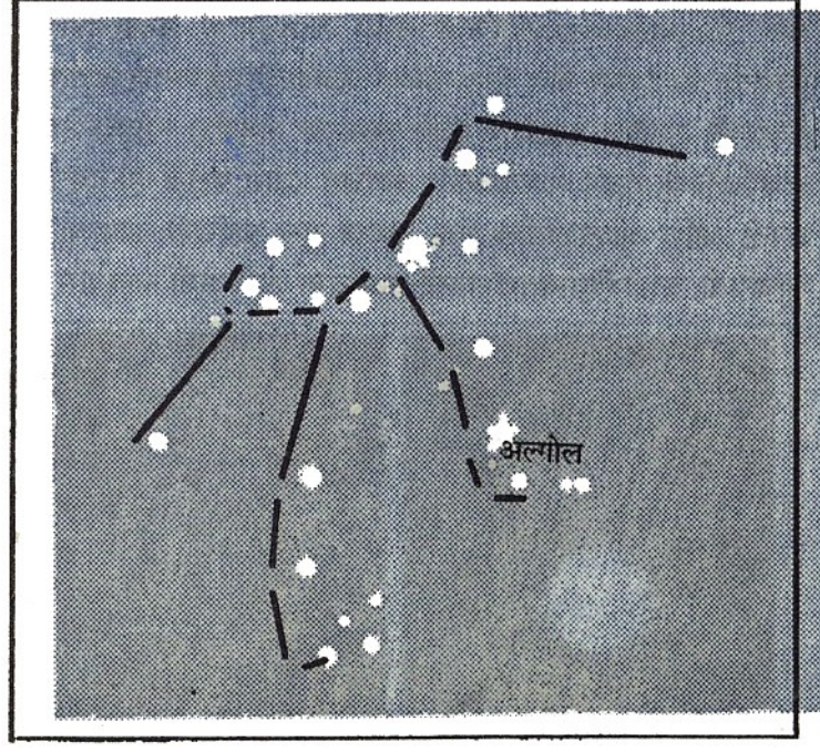
ययाती [Perseus] नक्षत्रामधील ग्रहणाधीन फेरफार होत असणारा तारा-अल्गोल
