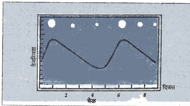
सिफीड तारे यांचा असा एक वर्ग आहे की त्यातील घटक विशिष्ट कालबद्धतेत ताऱ्यांची तेजस्विता कमी-अधिक झालेली दाखवित असतात.
