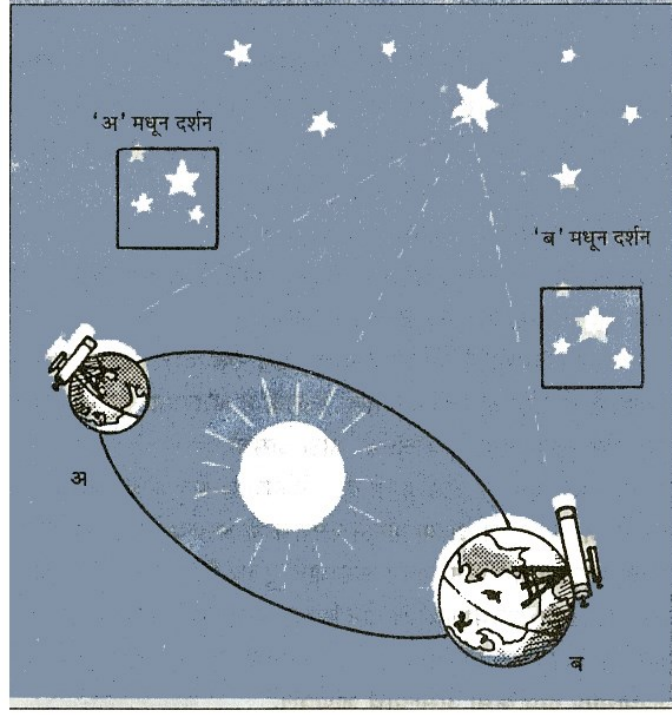
जर्मन खगोलशास्त्रज्ञ एफ. डब्ल्यू. बेसेल याने सहा महिन्यांच्या फरकाने दोन वेगवेगळ्या रात्री ताऱ्यांचे परीक्षण करून त्यांच्या पॅरेलॅक्स चे मोजमाप केले.
