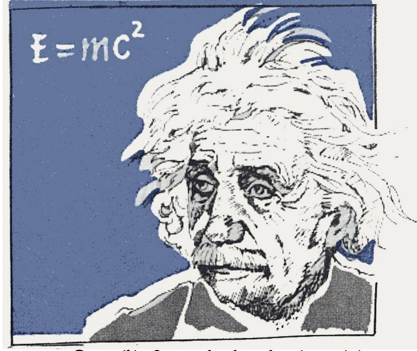
आण्विक ऊर्जेचे गुपित अल्बर्ट आइन्स्टाईन याने उघड केले.
