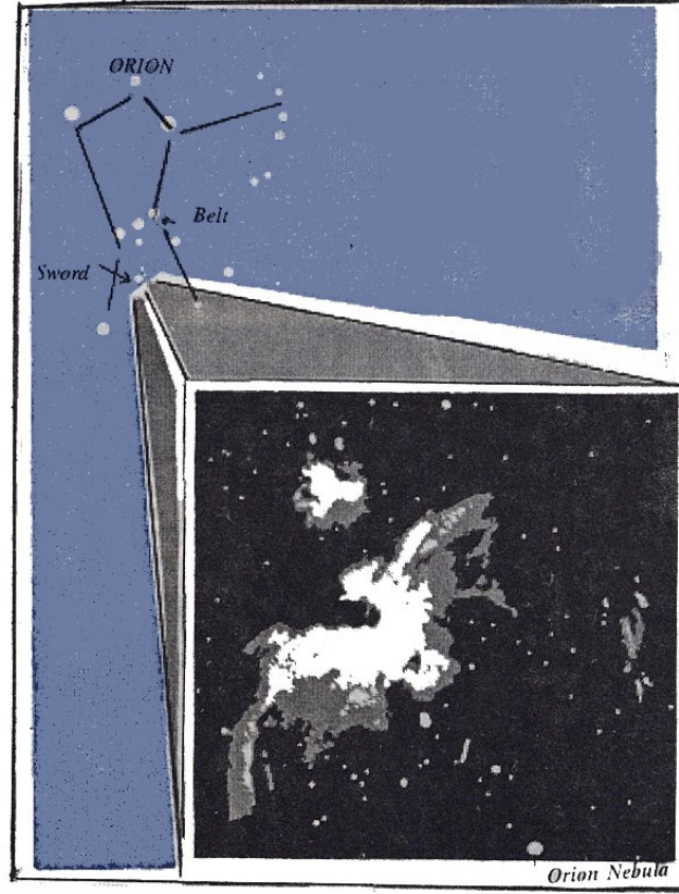
ताऱ्यांचे उगमस्थान. मृग नक्षत्रामधील ढगांचा पुंजका हे असे स्थान आहे की जिथे तारे नवीनपणे उदयास येत आहेत.
