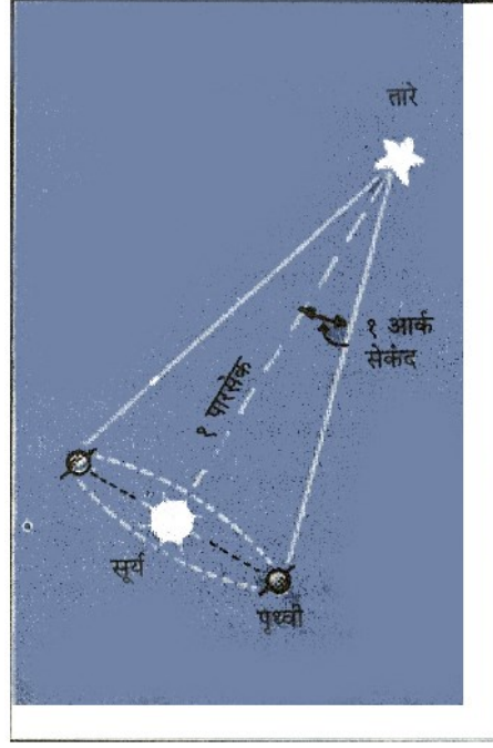
‘पारसेक’ – अंतरे मोजण्याची सोयिस्कर पद्धती
