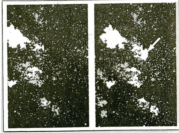
1987 च्या सुपरनोव्हाचे छायाचित्र. डावीकडील छायाचित्र विशाल मेगॅलान ढगांचे आहे, आणि सुपरनोव्हा दिसण्याच्या आदल्या रात्रीचे आहे. उजवीकडील छायाचित्रांत सुपरनोव्हाचा जन्म बाणाने दाखविला आहे.
