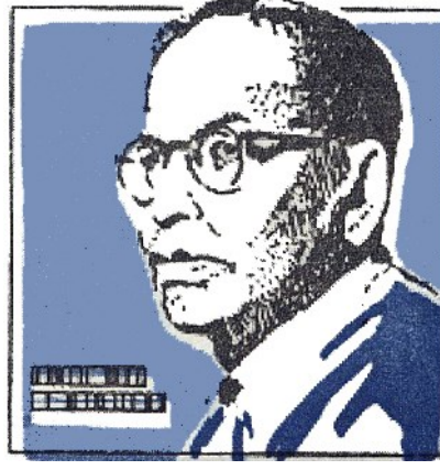
मेघनाद सहा यांनी ताऱ्यांच्या वर्णपटांचा अर्थ लावला.
