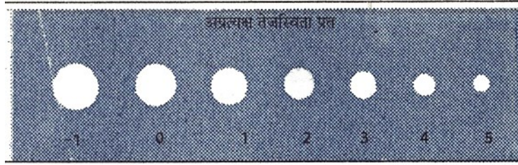
ताऱ्यांची तेजस्विता स्पष्ट करणारी पद्धत
