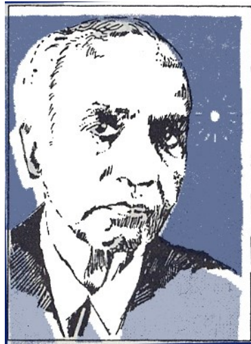
सुब्रह्मण्यम् चन्द्रशेखर यांनी श्वेत बुटके याची मर्यादा विशद केली.
