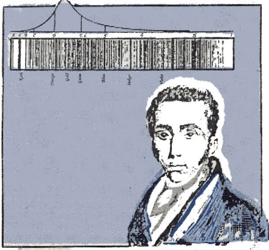
फ्रॉनहॉपर आणि त्याने शोधलेल्या काळ्या वर्णरेषा
