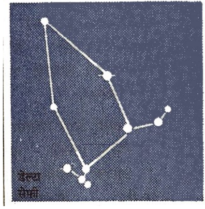
सेफ्यूस नक्षत्र – १७८४ मध्ये डेल्टा सेफ्यूस ताऱ्याचा शोध घेतला गेला
