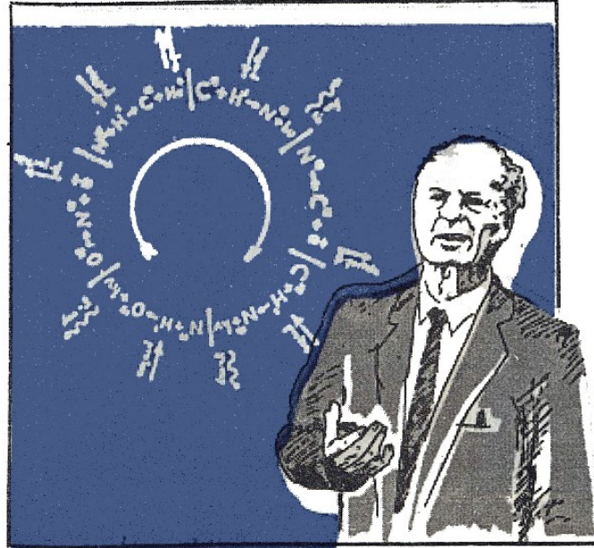
संपूर्ण आण्विक एकीकरणाची कल्पना हन्स बेथे याने समजण्यास सुलभ केली.
